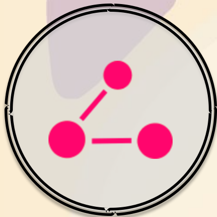
Visual DSL
